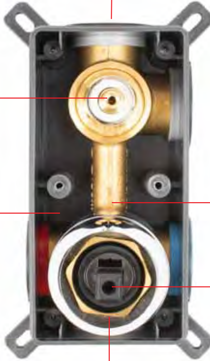
Levelling Scale For Easy Install Montaj Kolaylığı Sağlayan Terazi Sistemi
